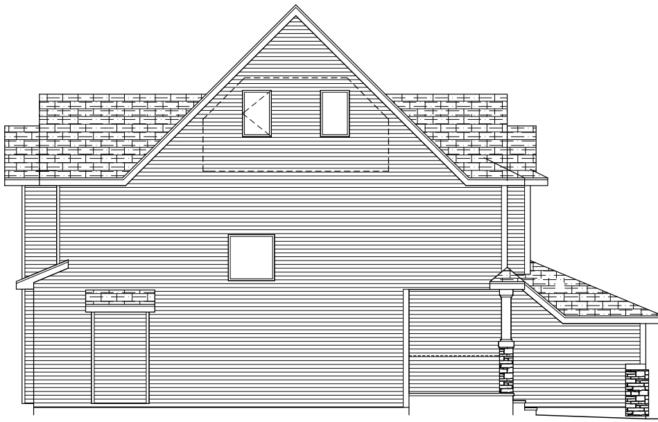
RIGHT ELEVATION "A"
