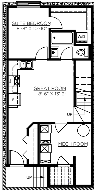
Optional Legal Suite 520 Sq Ft
