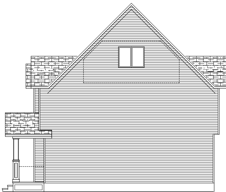
RIGHT ELEVATION "A"
